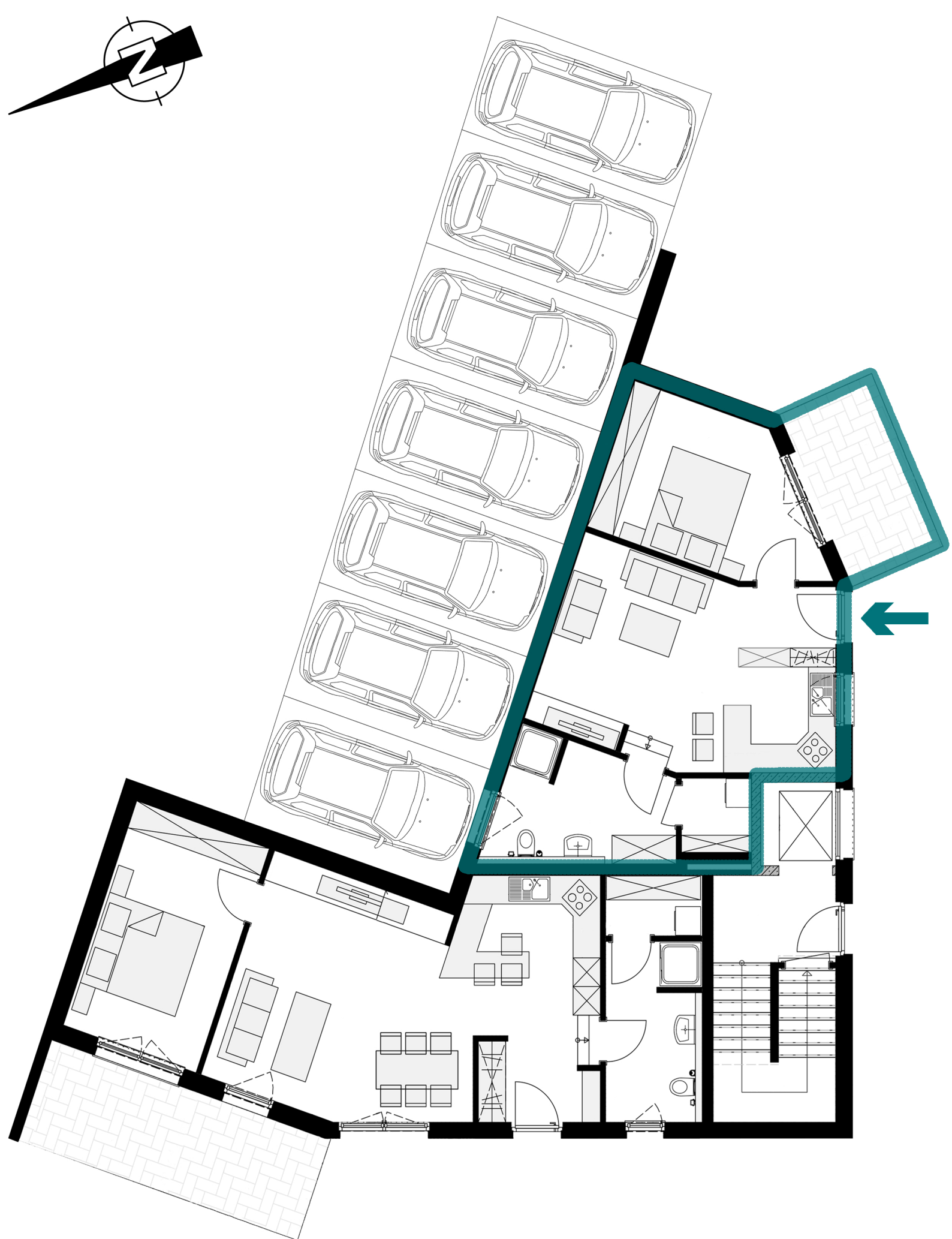
Osnabrück, Pottbäckerweg 2 Erdgeschoss, Whg. 2
