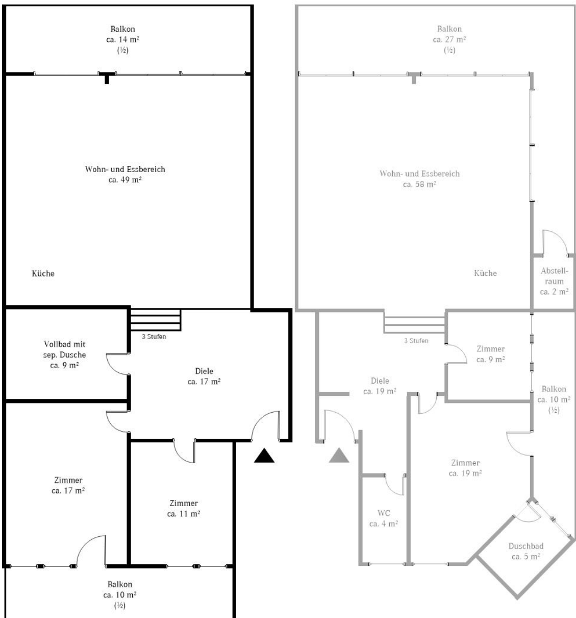
Hochparterre - Whg. 03 (Kaufoption Whg. 04)
