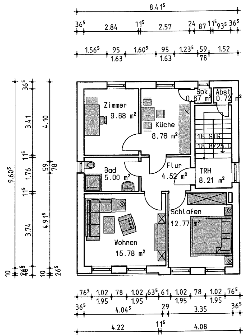
1. Obergeschoss
