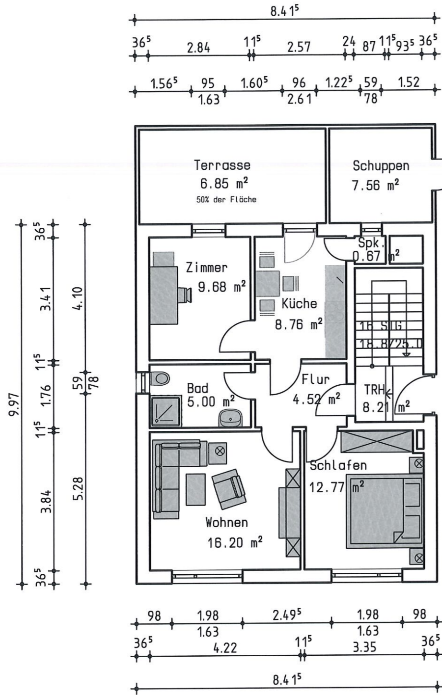
Erdgeschoss
