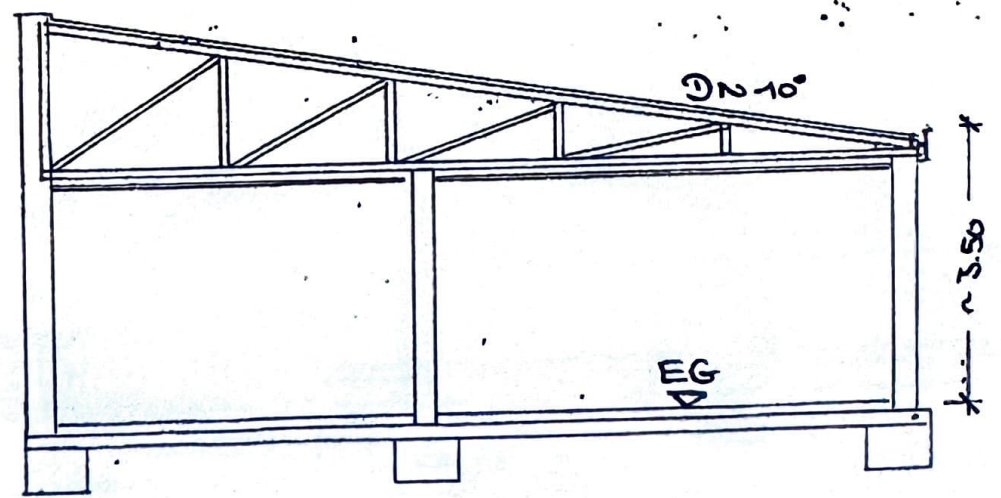
SCHNITT BB' M 1:100
