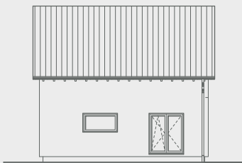
Ansicht Rechts
