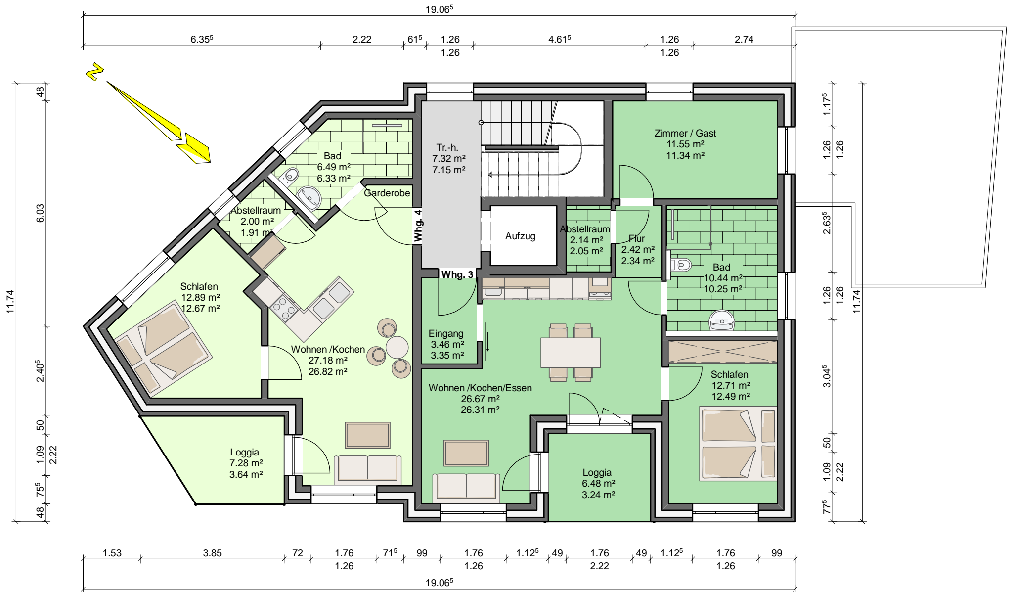
Obergeschoss 1
