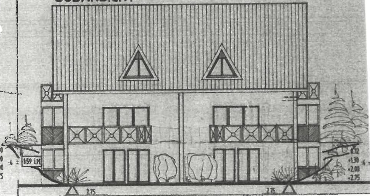
SÜDANSICHT
