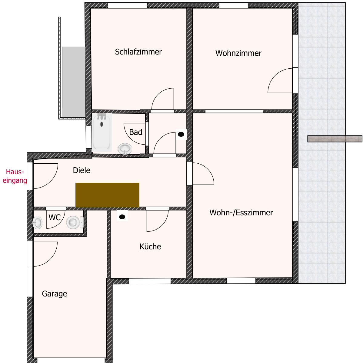
Grundriss Erdgeschoss (nicht maßstabsgetreu)
