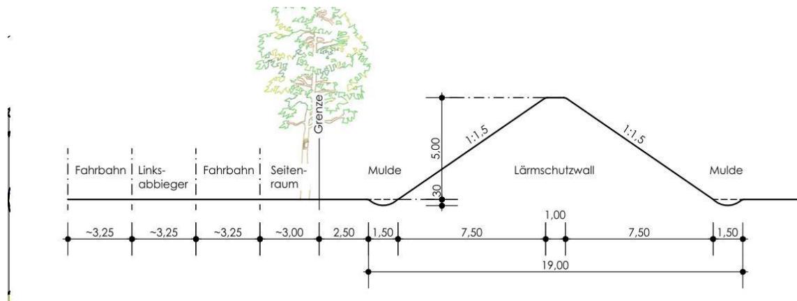
Abbildung 10: Querprofil Wallanlage L 190 6
