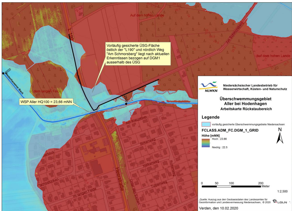
Abbildung 18: Verlauf vorläufig gesichertes Überschwemmungsgebiet 12
