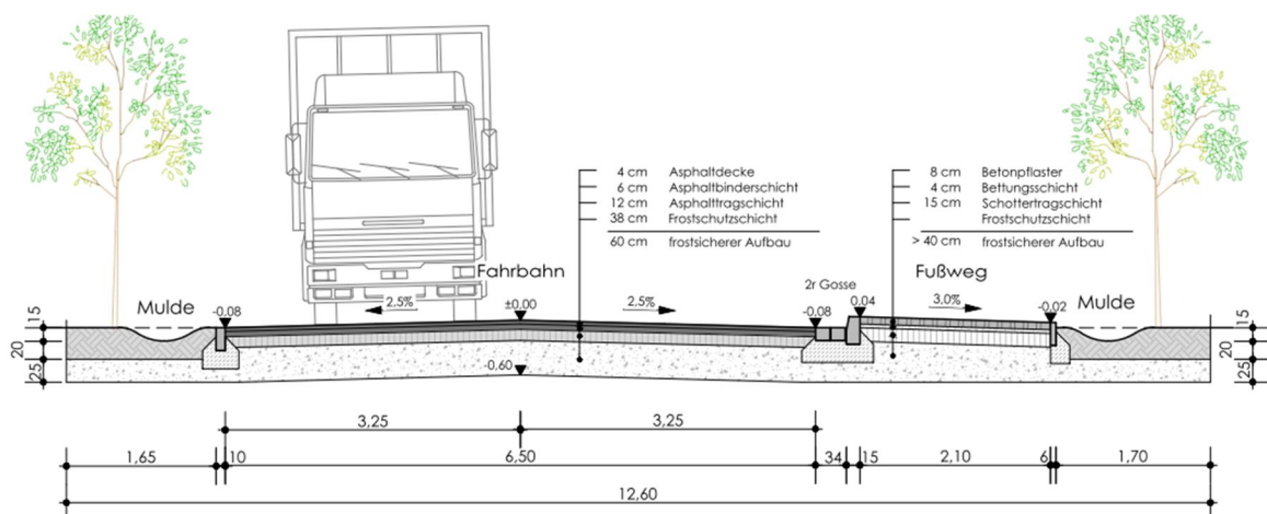
Abbildung 12: Querschnitt Planstraße C – Südrand des Plangebietes 8
