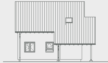
Ansicht Links
