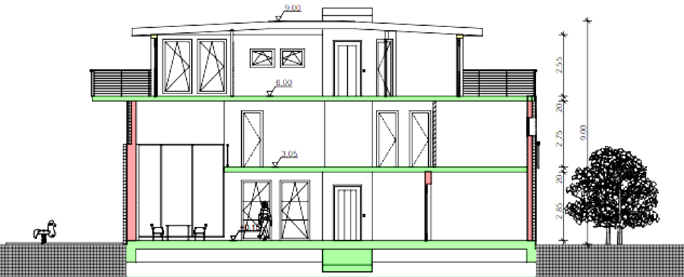
Schnitt D-D
