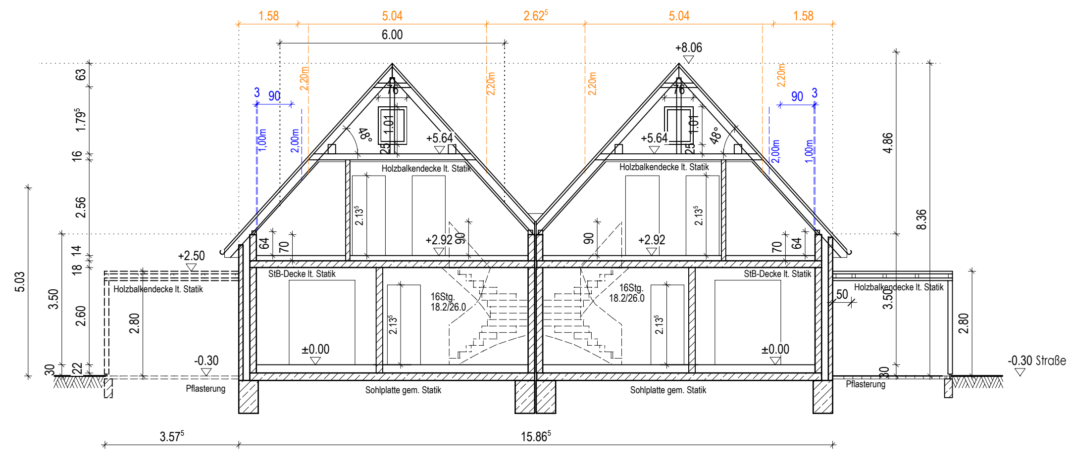
Schnitt A-A
