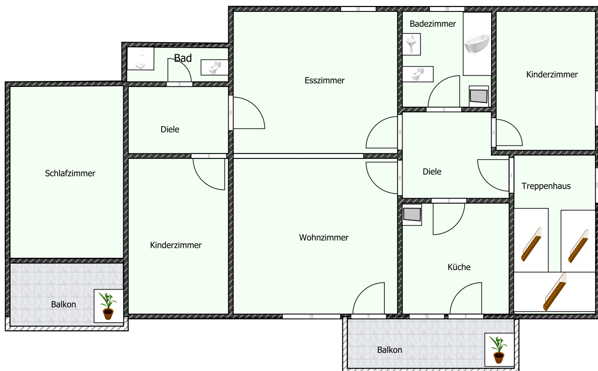
Grundriss Erdgeschoss (nicht maßstabsgetreu)
