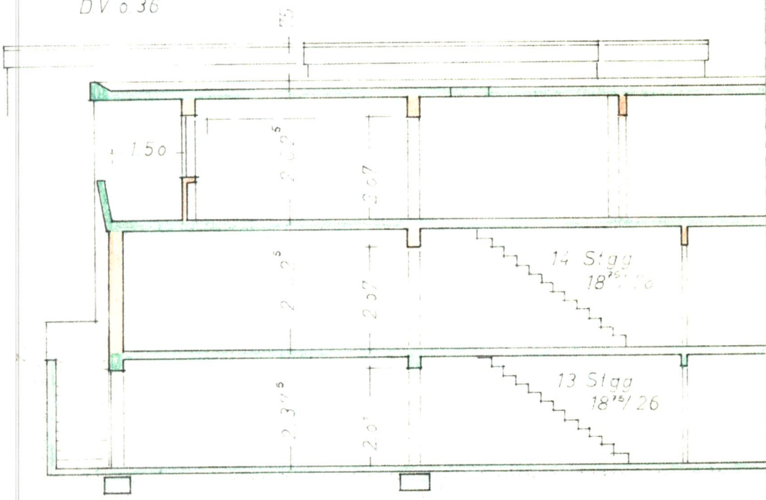
Schnitt a-b
