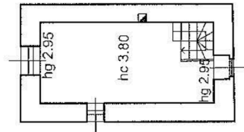
PIANO TERZO
