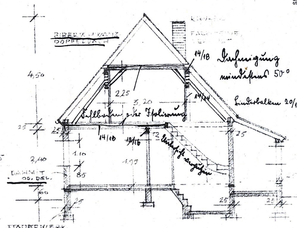
SNITT A-B
