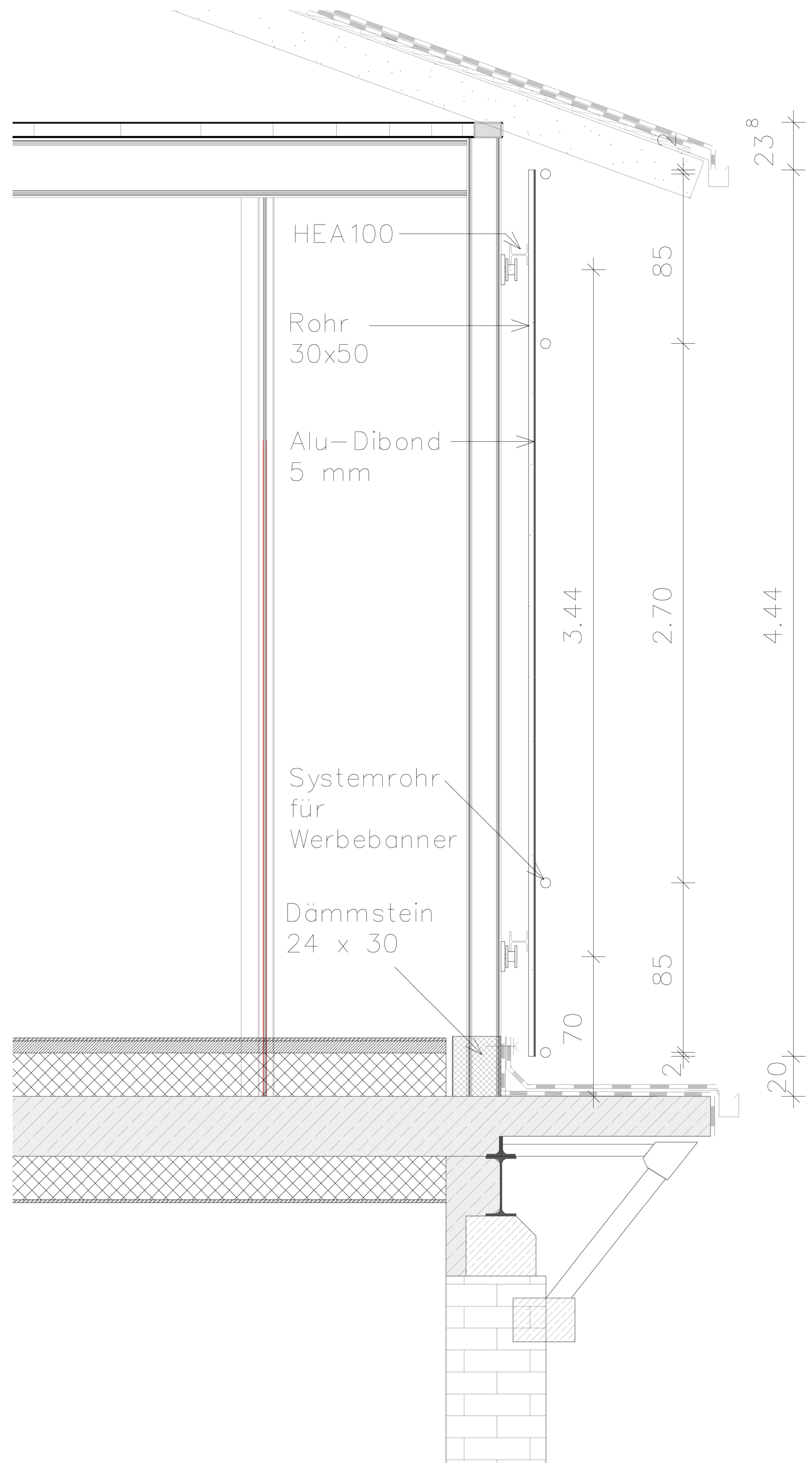
Werbeträger Schnitt 1:25
