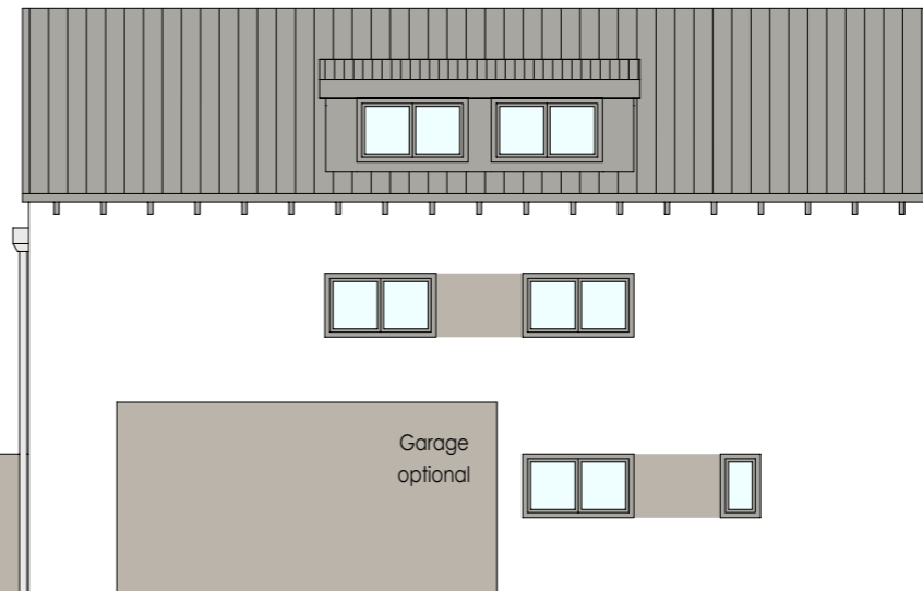
Nordostansicht
