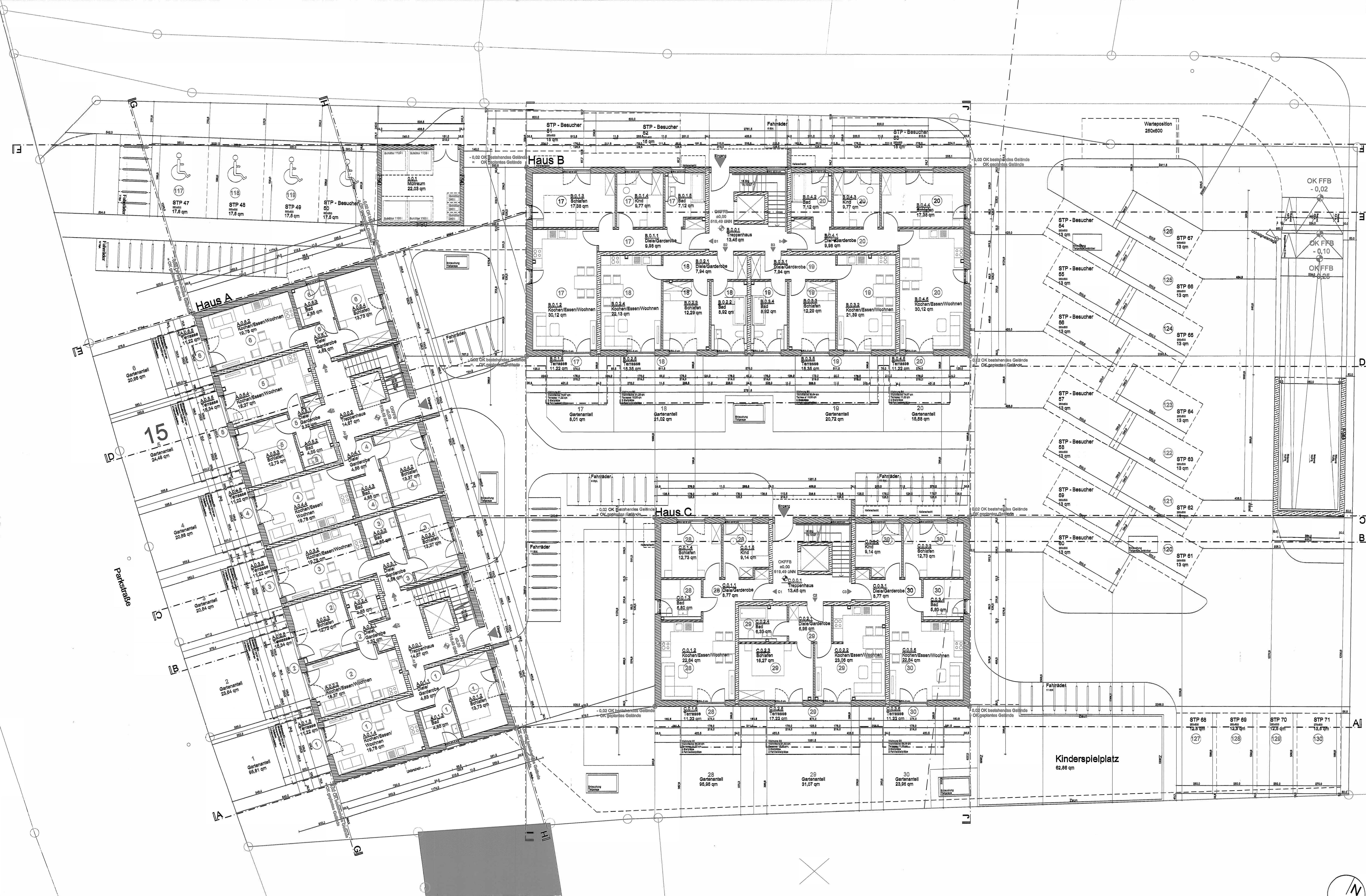
Edgeschoss M1:100
