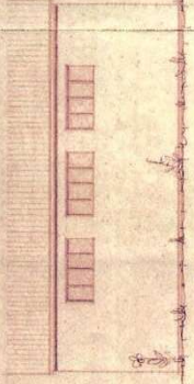
Öst-Ansicht
