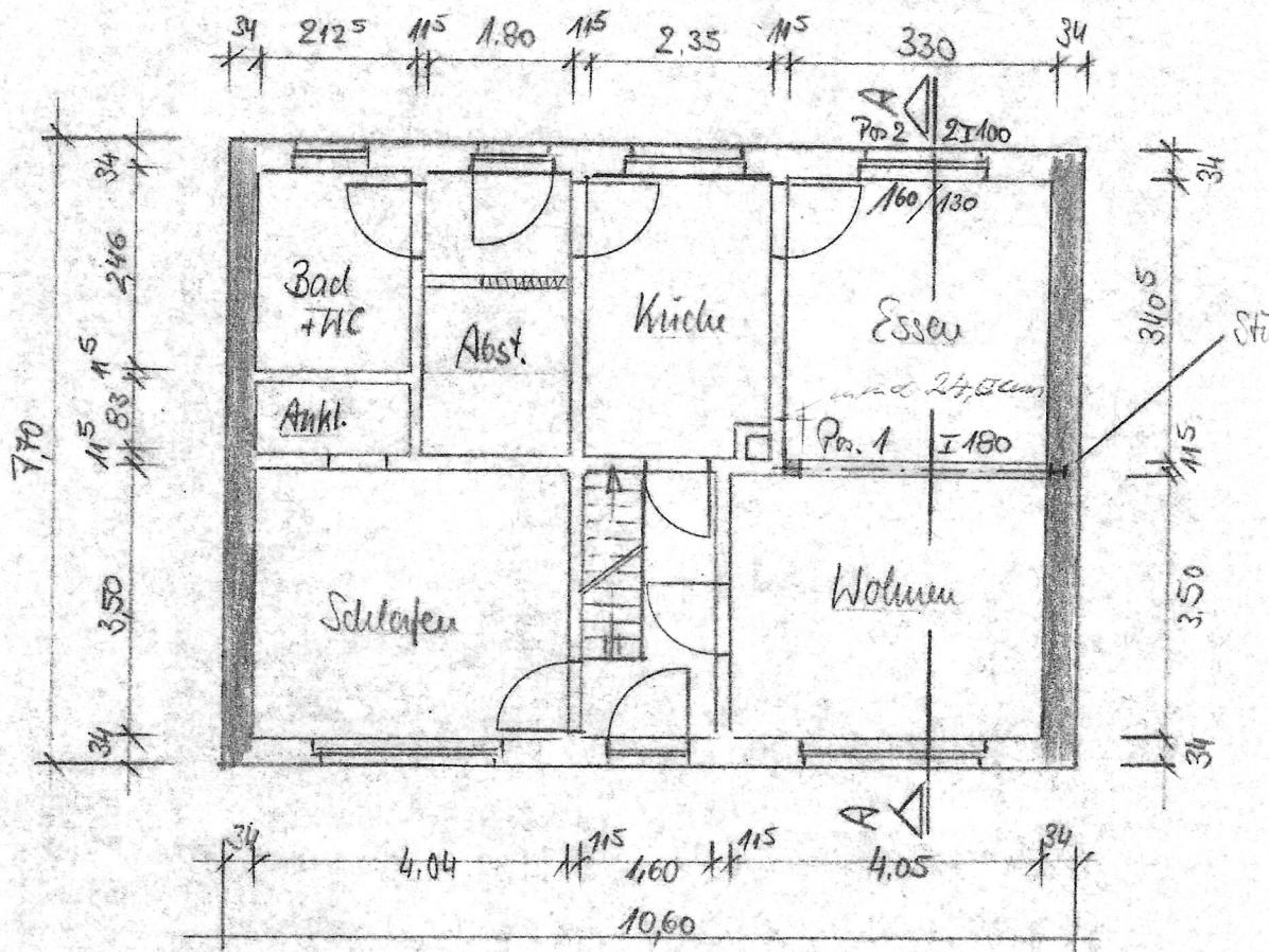
Grundriß = EG
