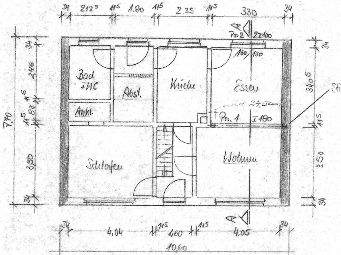
Grundriß = EG
