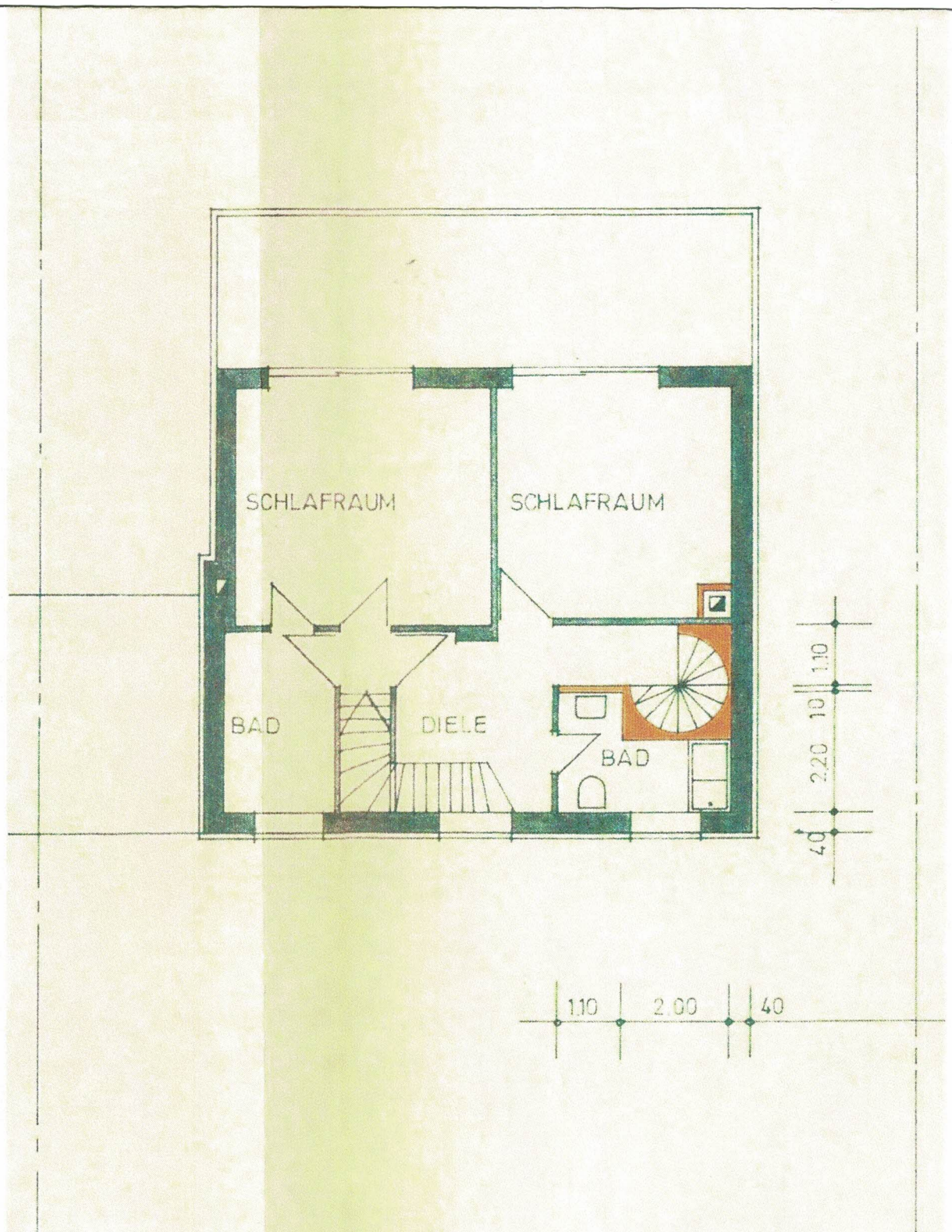
GRUNDRISS OBERGESCHOSS
