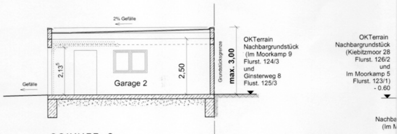
SCHNITT C
