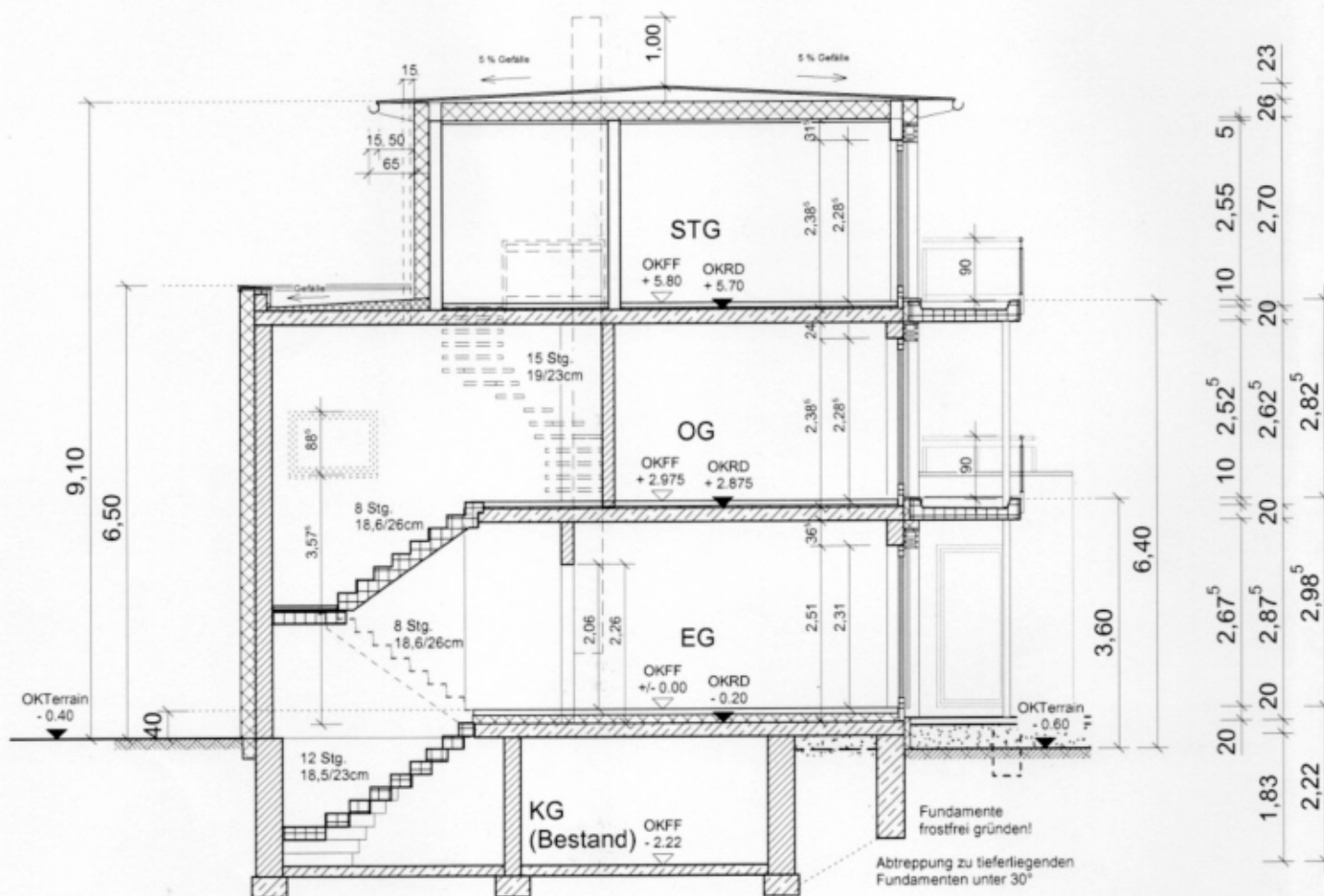
SCHNITT A
