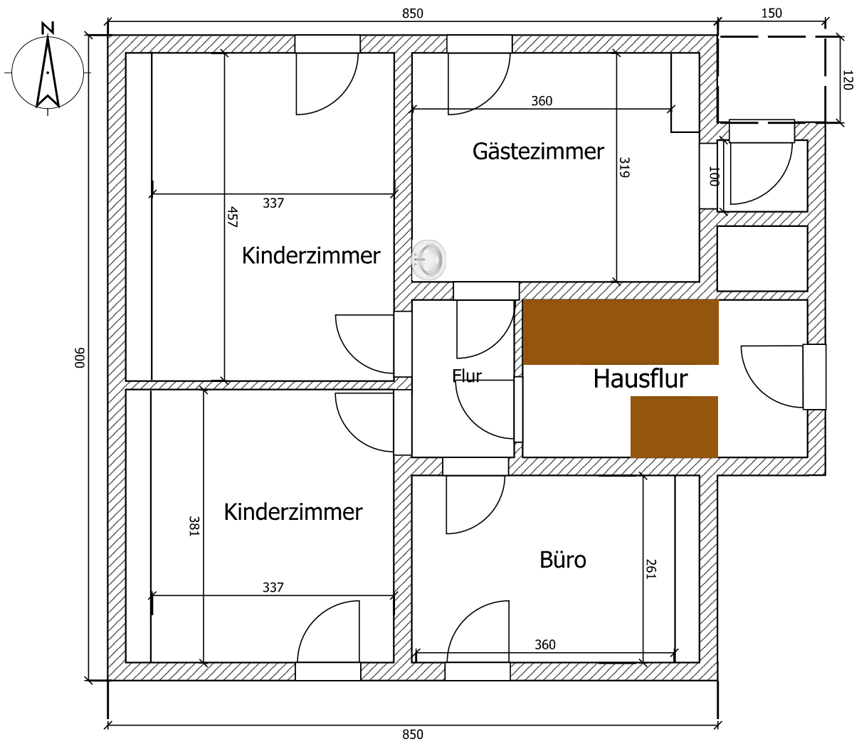
Dachgeschoss
