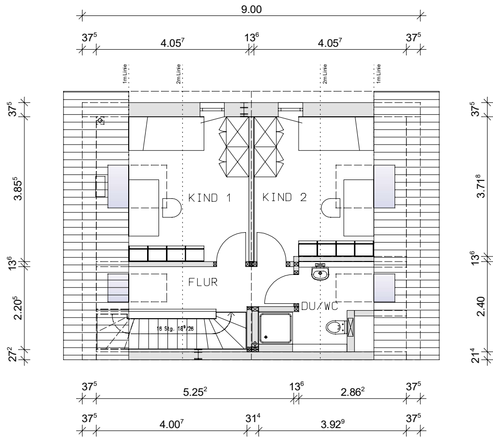
Grundriss Dachgeschoss M 1:100
