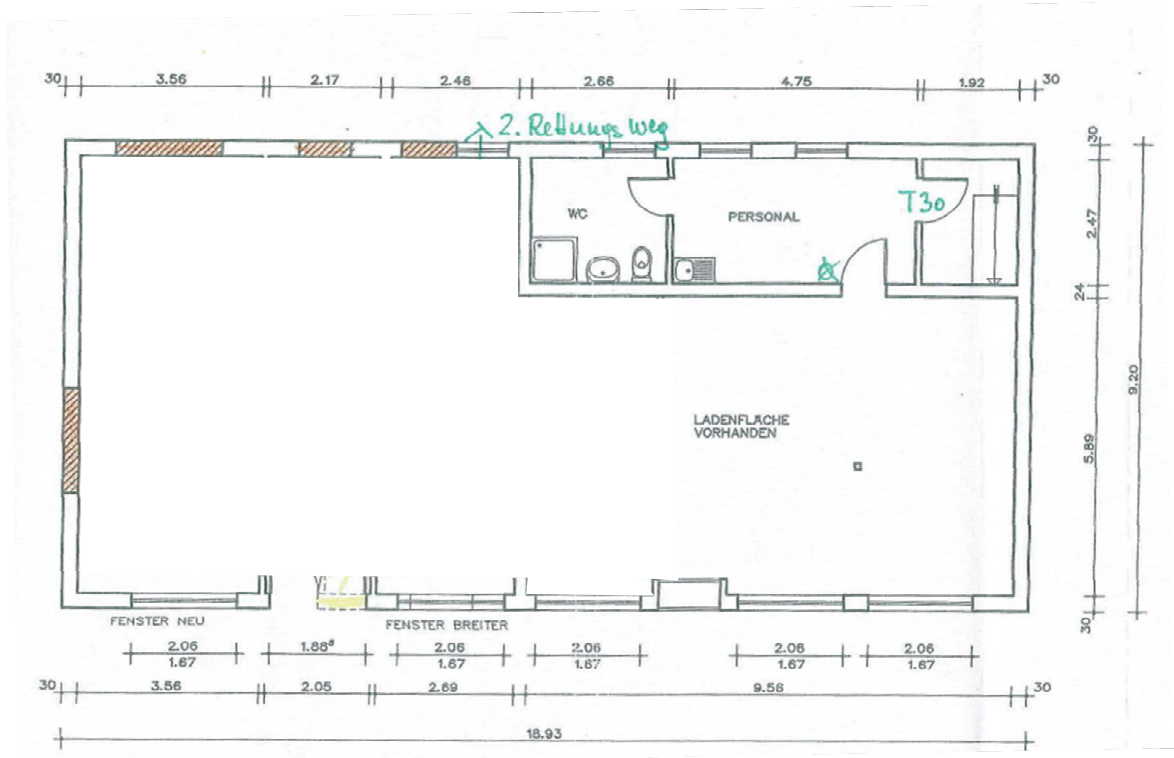
Grundriss Erdgeschoss
