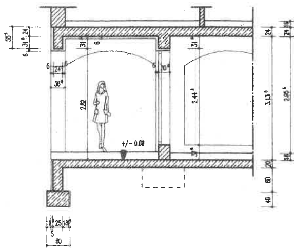
SCHNITT C-C M = 1:50
