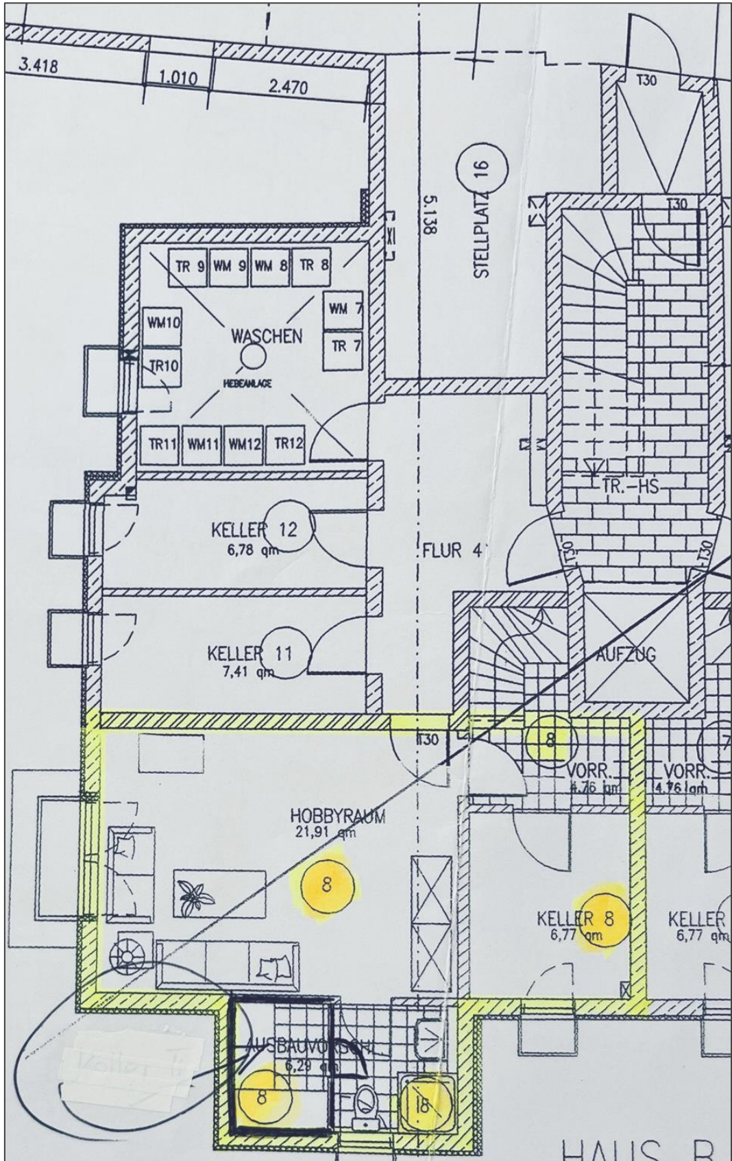
Grundriss UG
