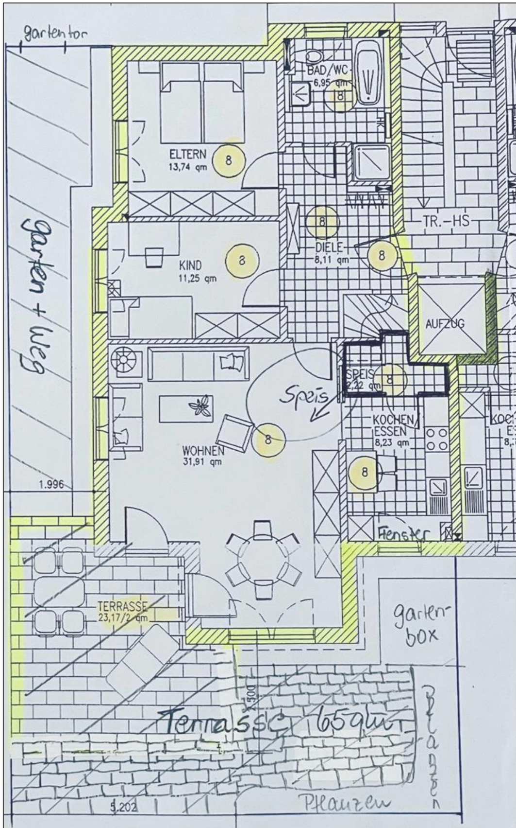
Grundriss EG
