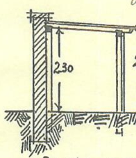
SNITT C-D
