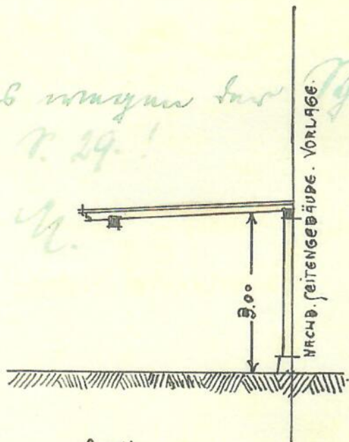
SNITT A-B.
