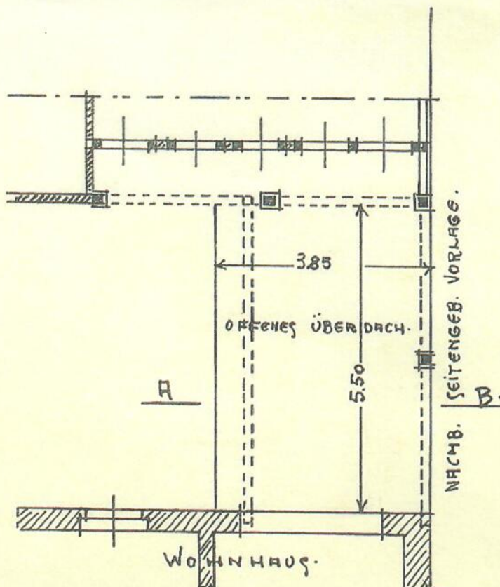
GRUNDRISS DES ÜBERDACHES.
