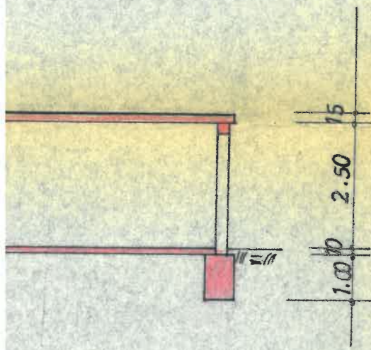
Schnitt a-a
