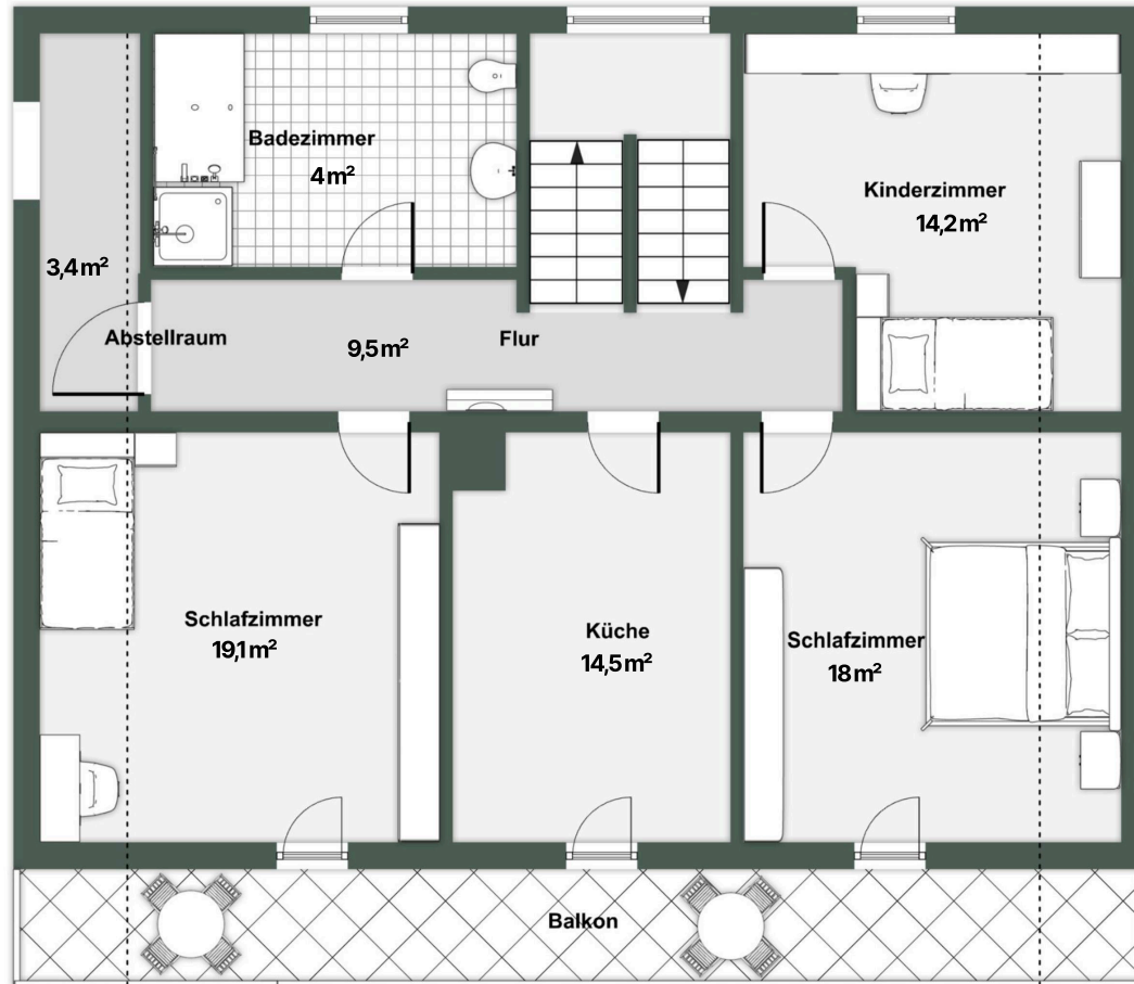
Obergeschoss
