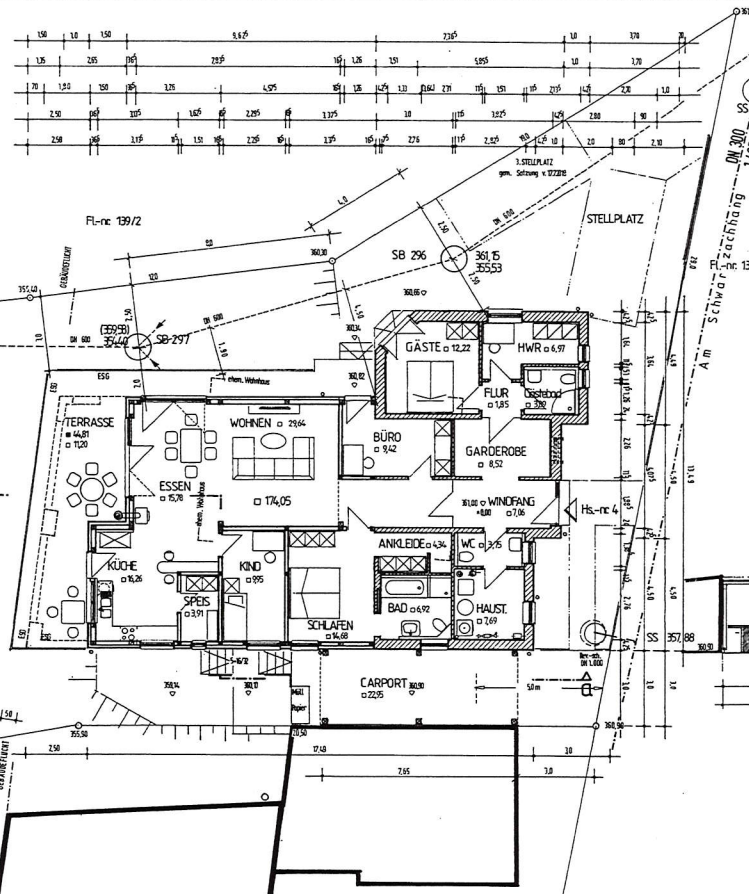
GRUNDRISS UNTERGESCHOSS
