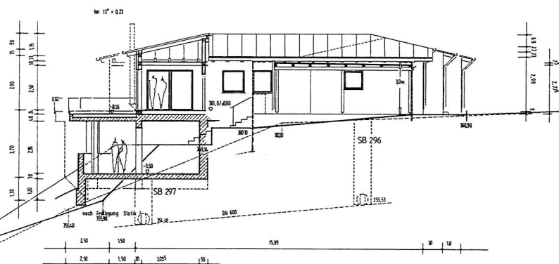
SCHNITT a-a 1/100
