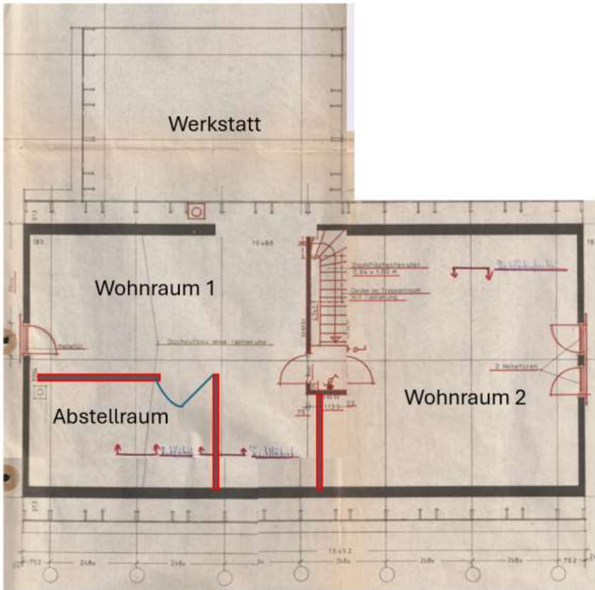
Grundriss Dachgeschoss
