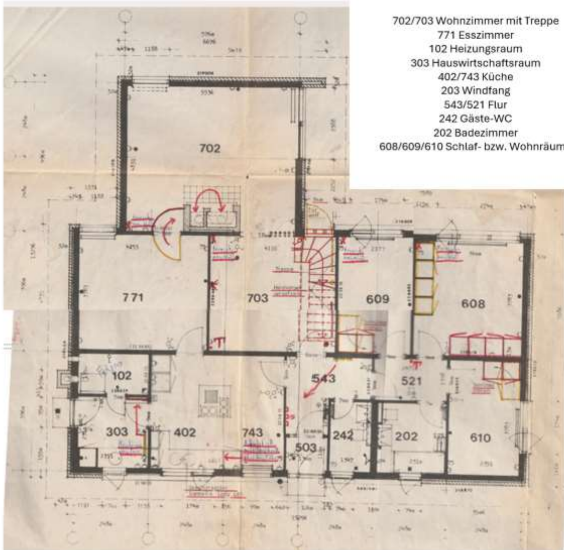
Grundriss Erdgeschoss
