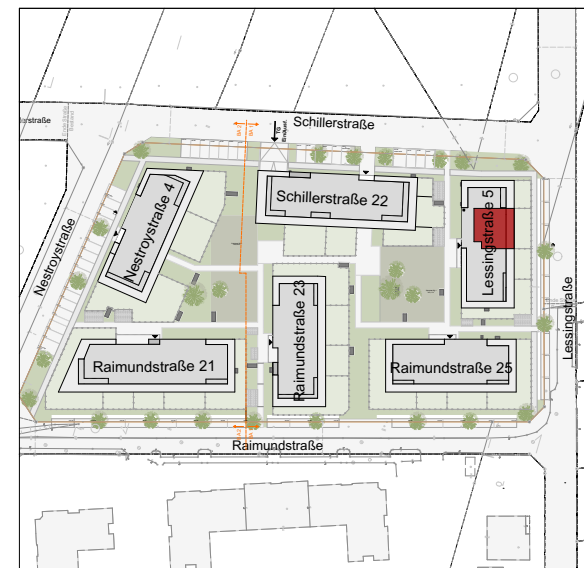
Lageplan
