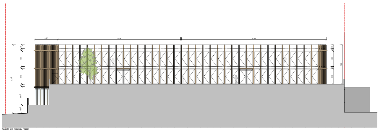
Ansicht Ost (Neubau Plaza)
