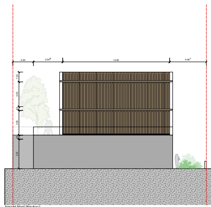
Ansicht Nord (Neubau)
