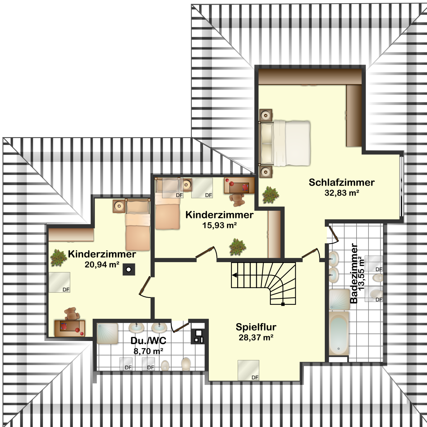
Obergeschoss
