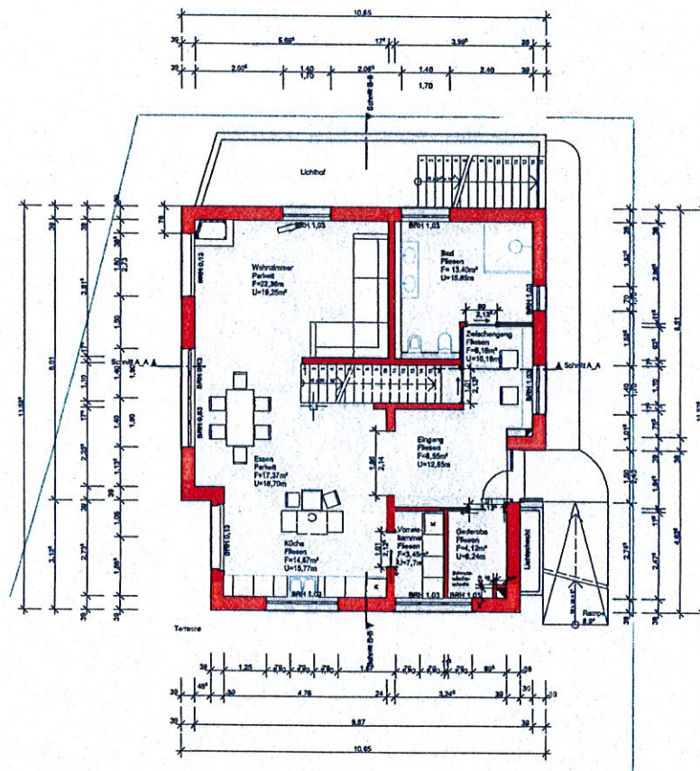
Erdgeschoss
