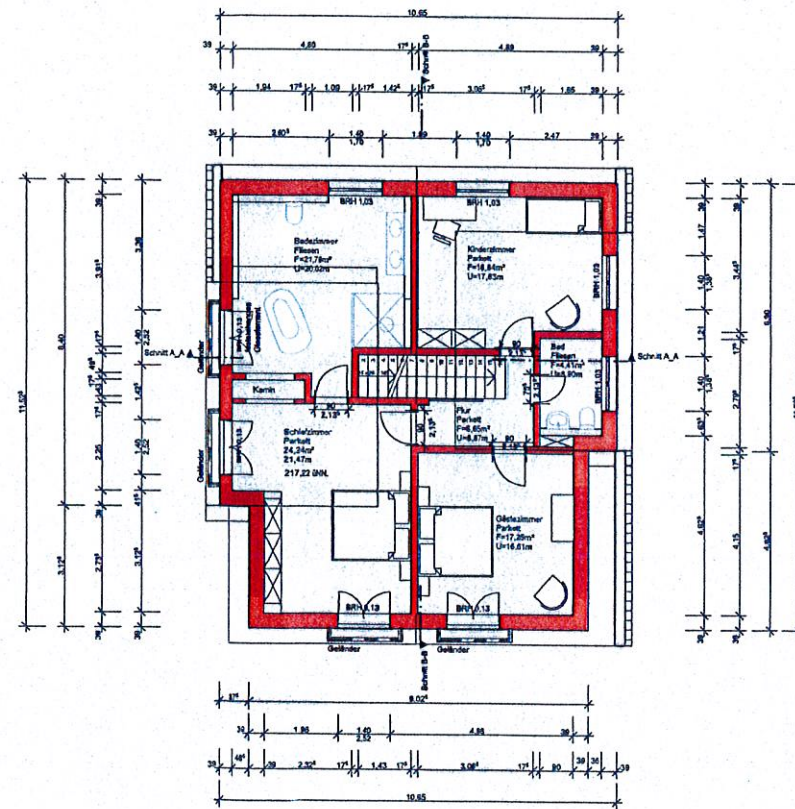
Dachgeschoss
