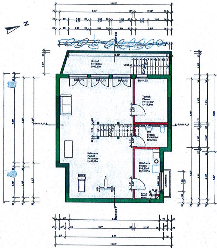
Kellergeschoss
