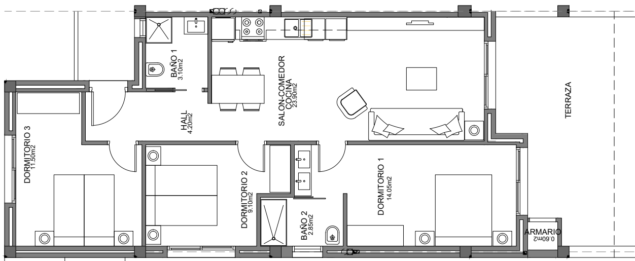
Planta Primera
