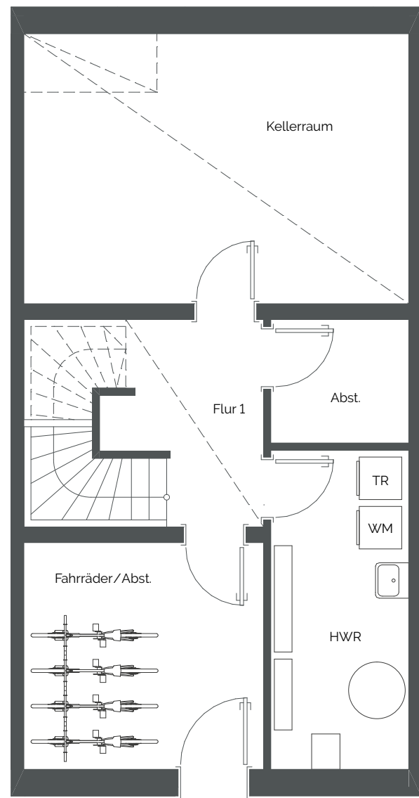
Kellergeschoss
