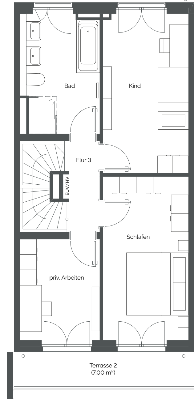
1. Obergeschoss
