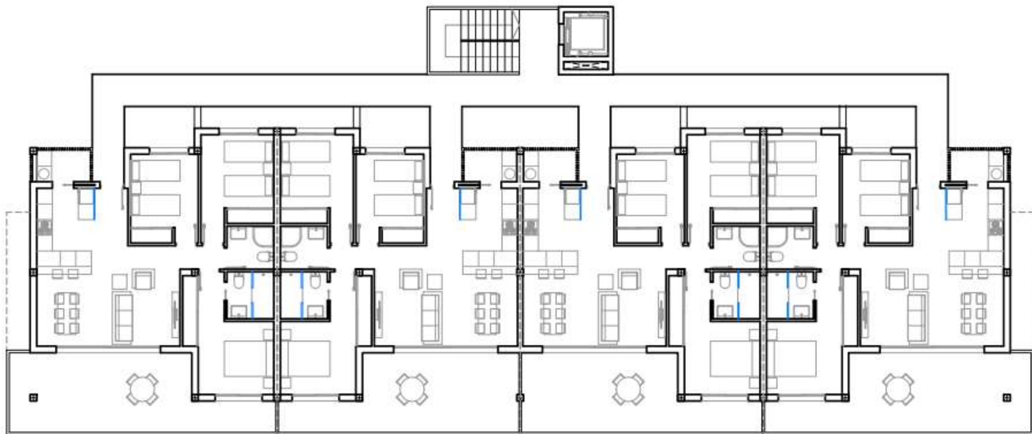
PLANTA PRIMERA
