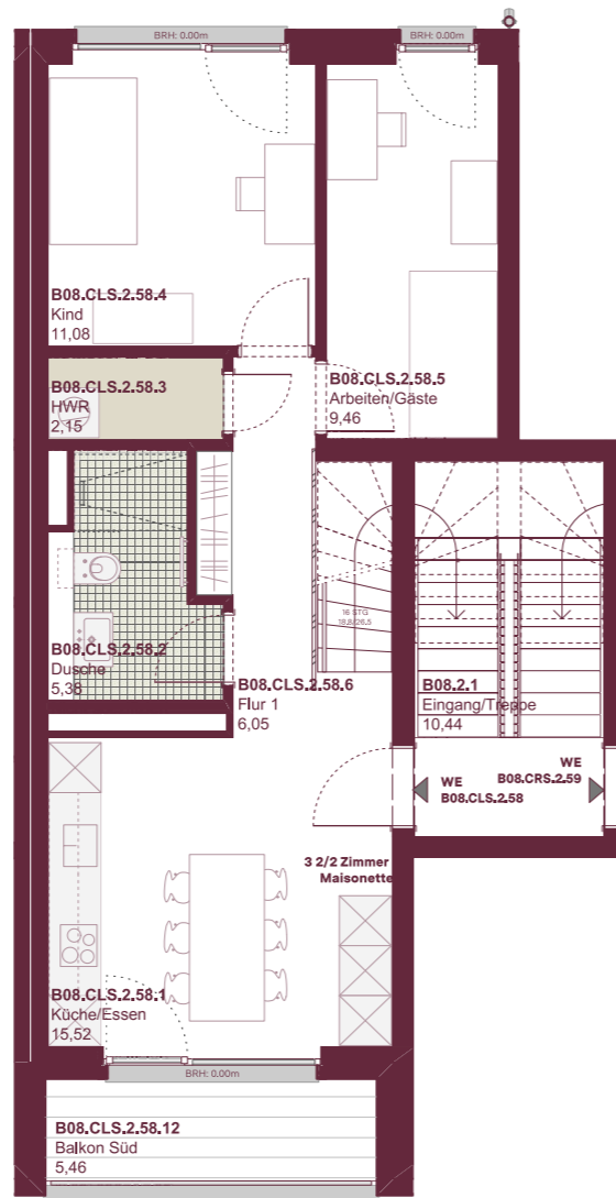
Grundriss 2. Obergeschoss M 1:100
