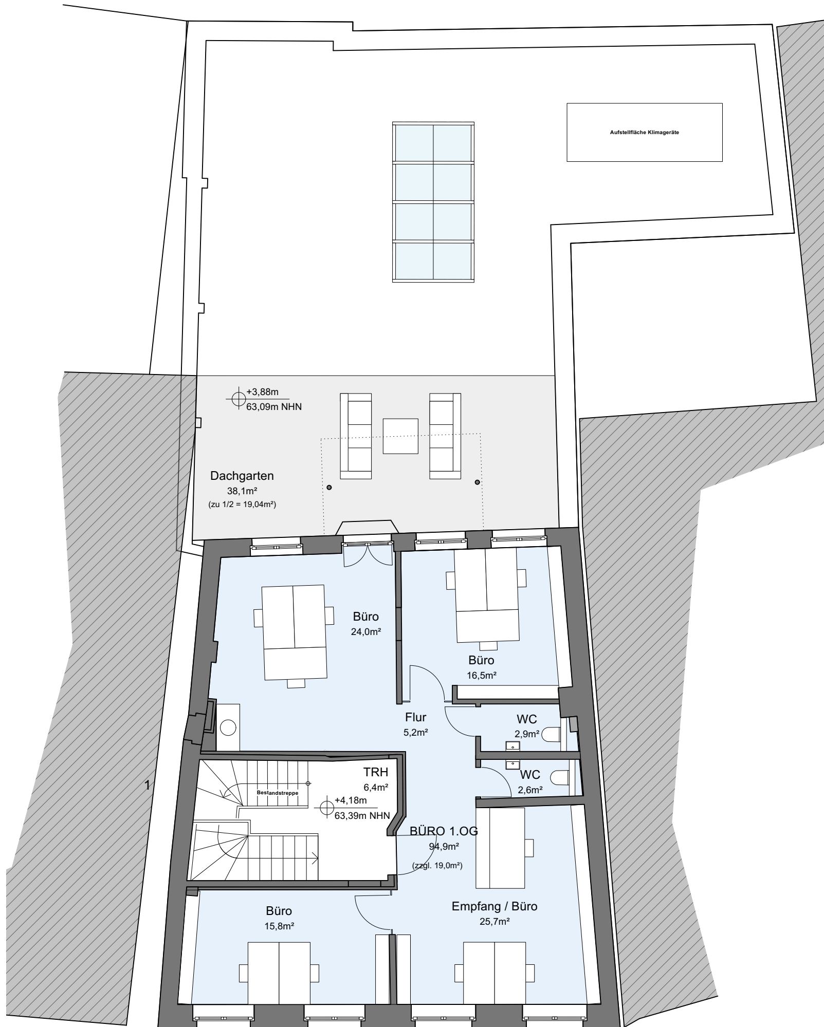
Grundriss 1.OG
