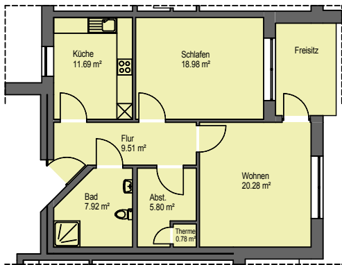
Nr. 17 EG WHG 3
