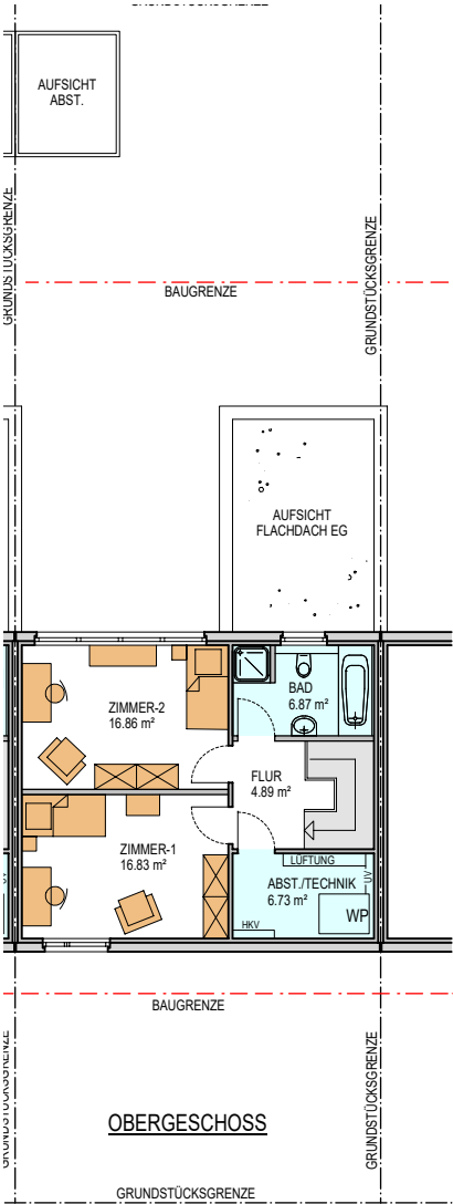
Mittelhaus Grundriss Obergeschoss 2 Zimmer
