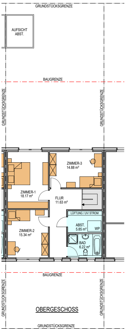
Mittelhaus Grundriss Obergeschoss 3 Zimmer
