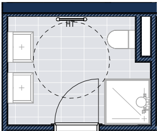
VARIANTE BAD 1
