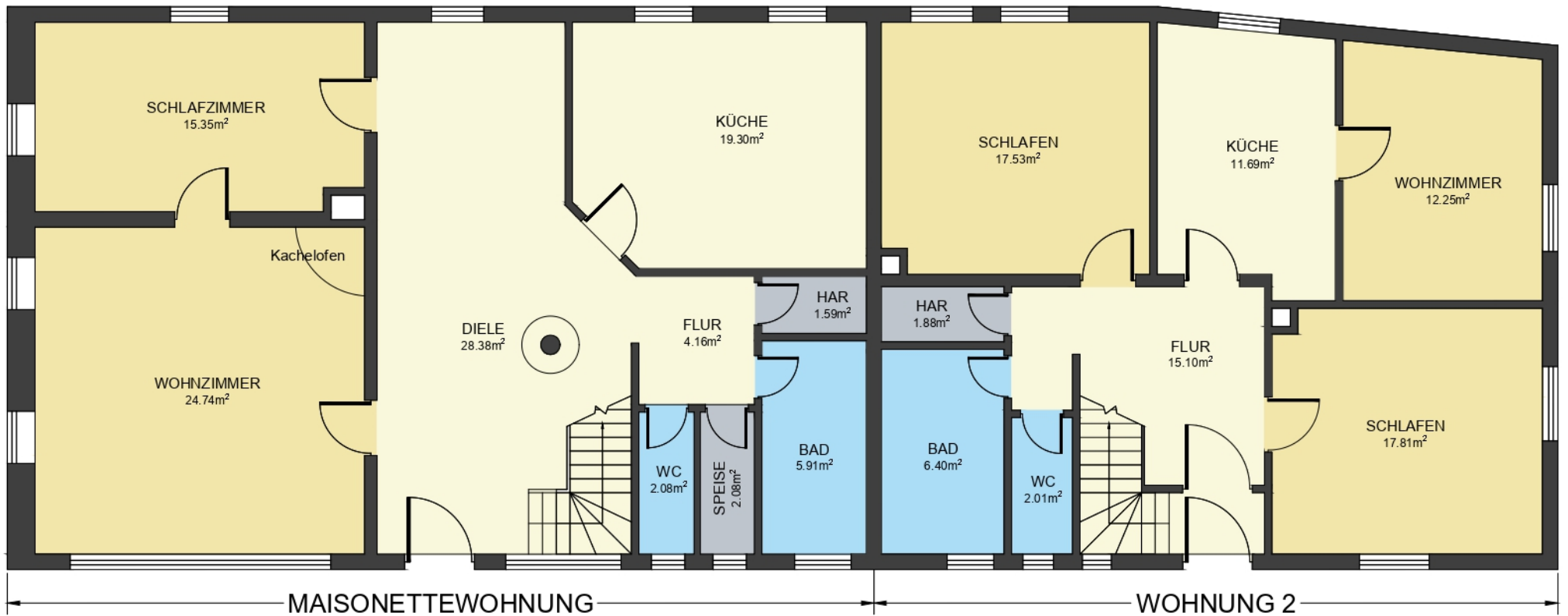
GRUNDRISS ERDGESCHOSS
