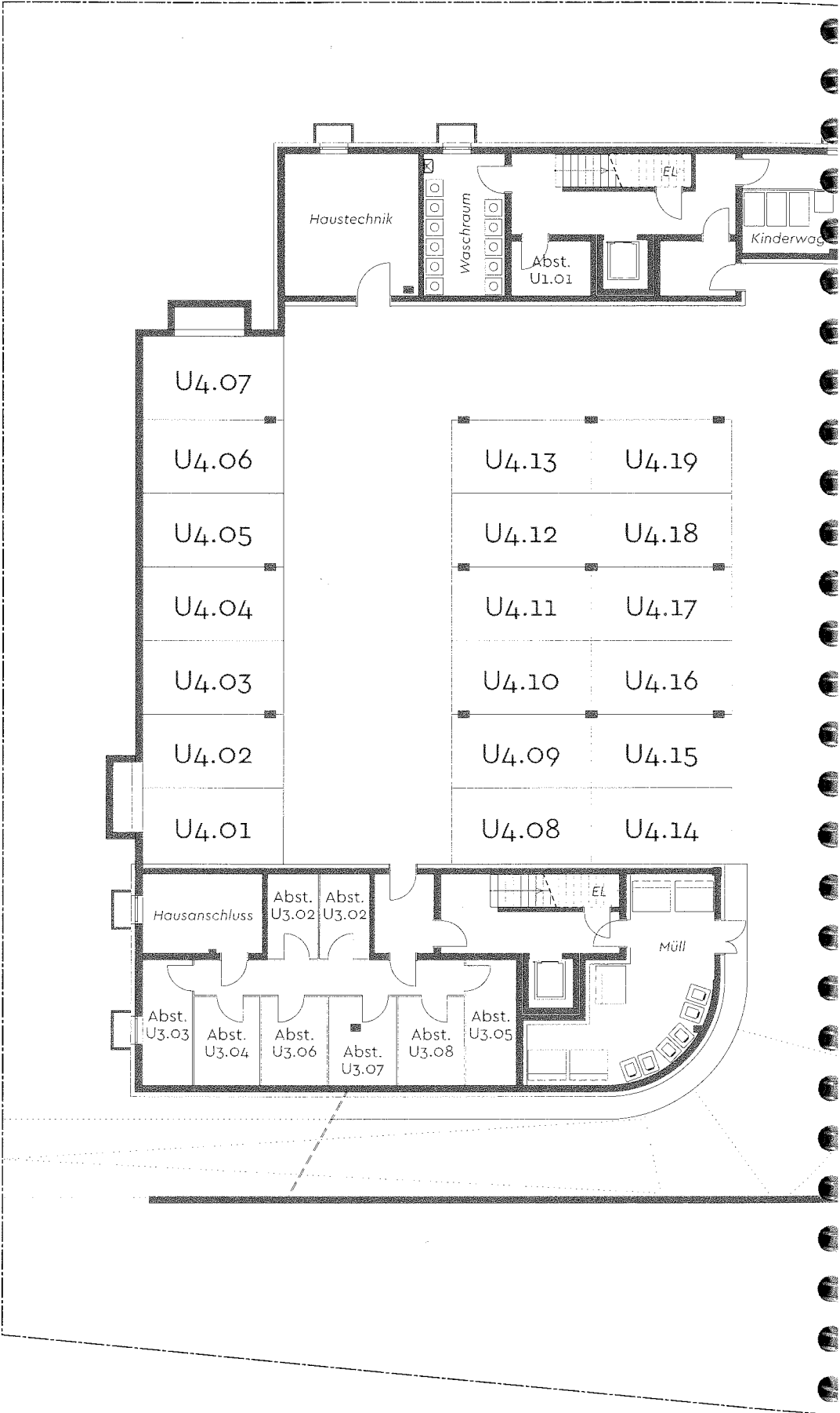
Untergeschoss | Tiefgarage
