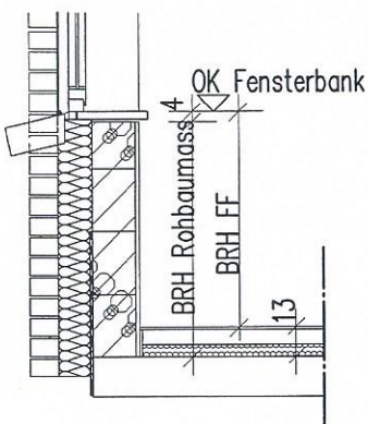
Detail Fenster Brüstungshöhen
