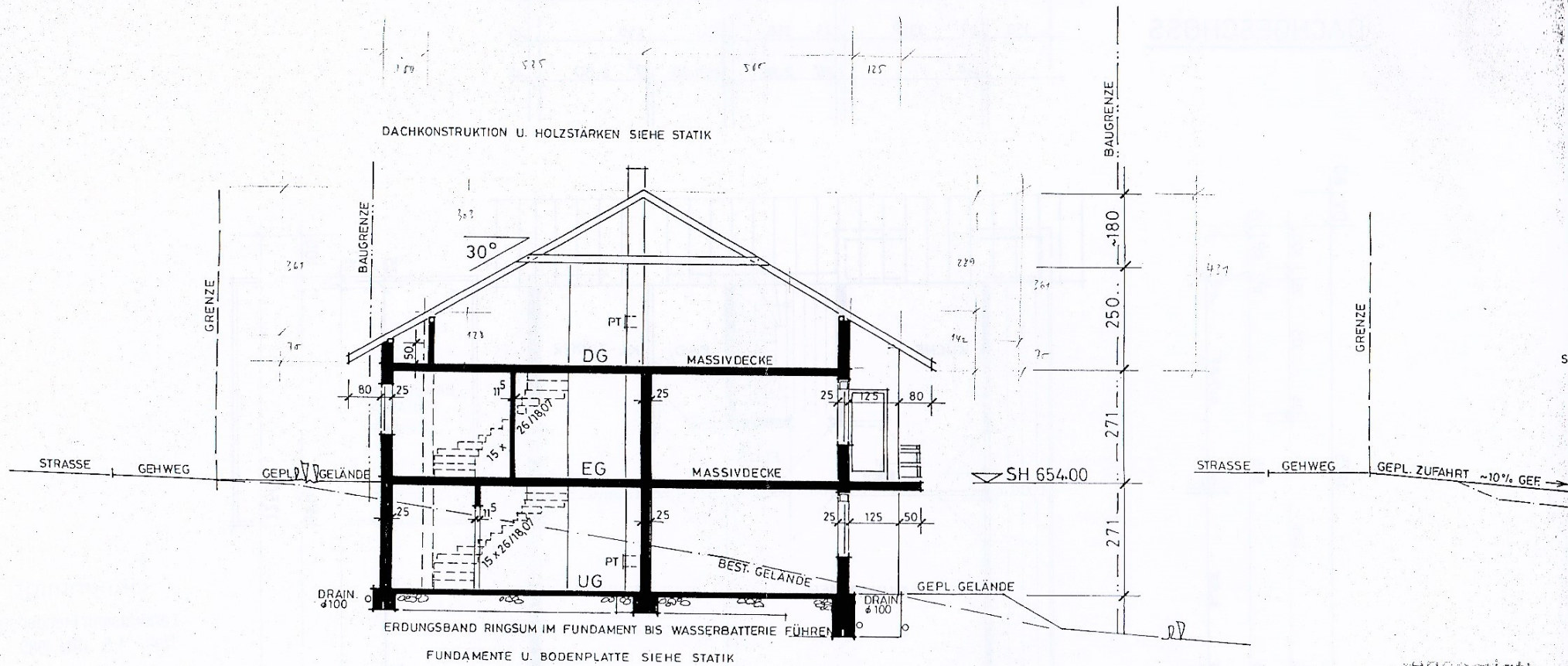
SCHNITT A-B
