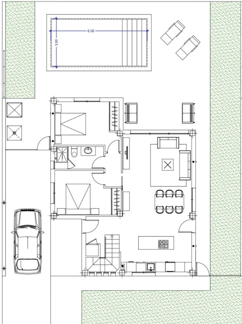
PLANTA BAJA
